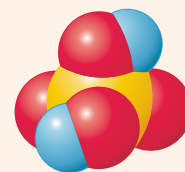
\text{H}_2\text{SO}_4
