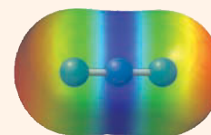
Azide ion
