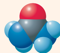
Urea
