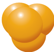
P 4
