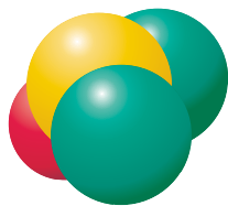
\text{SOCl}_2
