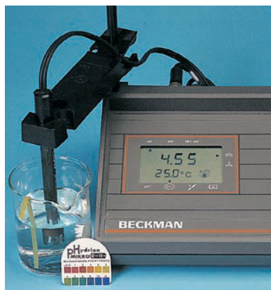
NH 4 Cl
