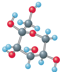
Fructose
