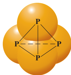
P 4
