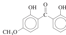
Oxybenzone
