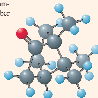
Camphor
