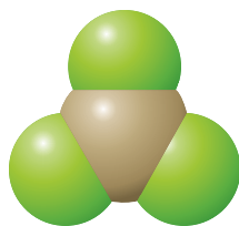
BF 3
