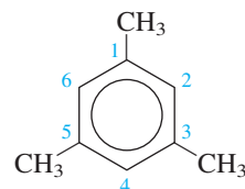
1,3,5-Trimethylbenzene
