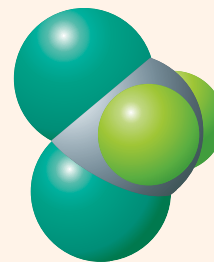
\text{CCl}_2\text{F}_2
